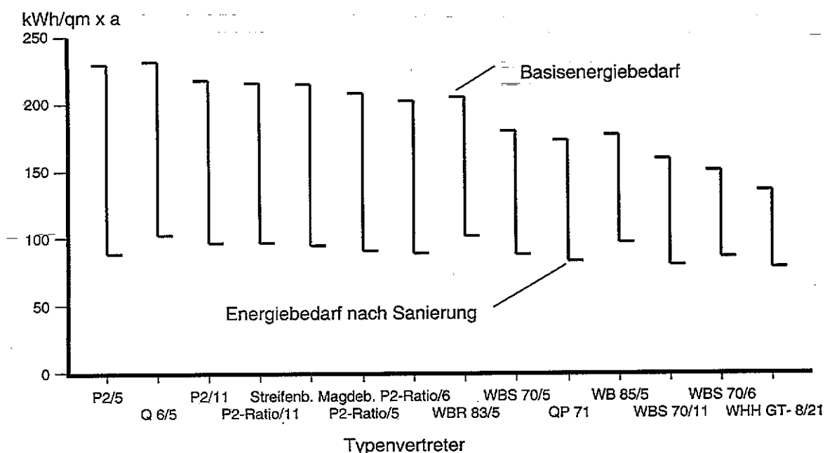
Jährlicher Heizenergiebedarf vor und nach der Realisierung energiesparender Maßnahmen
