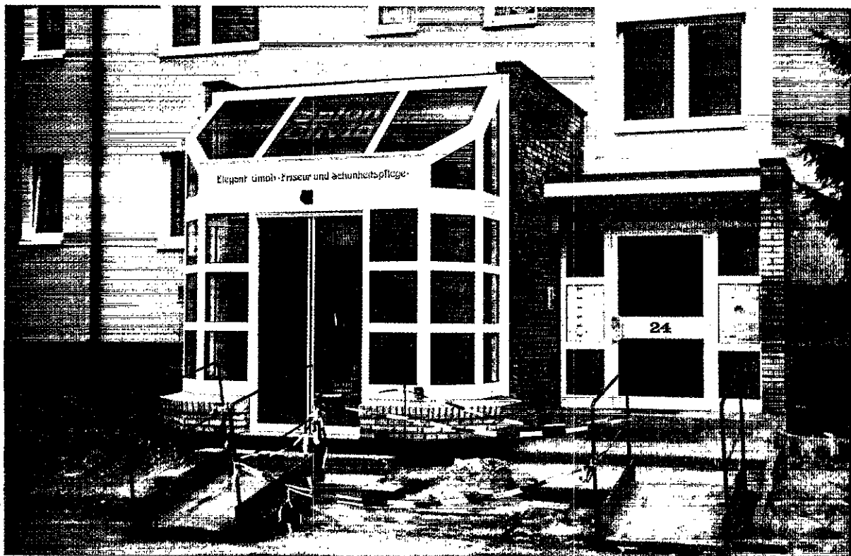
Zusätzliches Wärmedämmsystem, neuer Hauseingang und ein kleiner Friseursalon im Erdgeschoß
