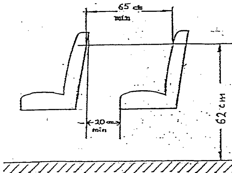
Abbildung 12b Abstand zwischen den Sitzen (siehe 7.7.8.4.1 b)
