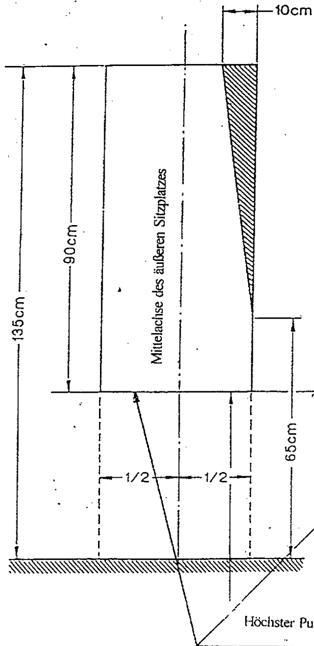
Abbildung 15 ZULÄSSIGES HERVORSTEHEN EINES BÜGELS DES FAHRZEUGAUFBAUS (siehe 7.7.8.6.3.2)
