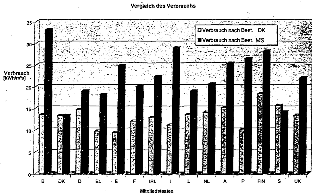
Abb. 3: Energieverbrauch in den Mitgliedstaaten entsprechend ihren geltenden Vorschriften für Gebäude im Vergleich zum dänischen Modell, unter Berücksichtigung klimatischer Unterschiede 18 19
