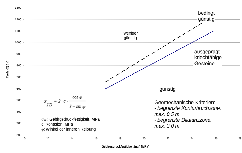
Abbildung 5-5: Maximal mögliche Endlagerteufe in Abhängigkeit von der Gebirgsdruckfestigkeit für Festgesteine mit ausgeprägt kriechfähigem (duktilem) Materialverhalten [nach LUX 2002 13 ]
