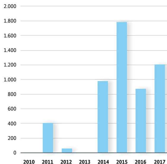
Abbildung 3: Jährlicher Leistungszubau in MW, Windenergie auf See seit 2010
