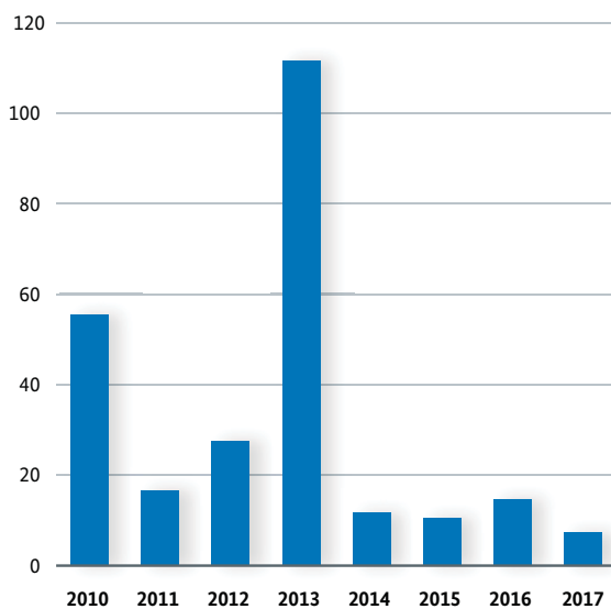
Abbildung 5: Jährlicher Leistungszubau in MW (netto, Neuinbetriebnahme, reaktivierte und ertüchtigte Anlagen), Wasserkraft seit 2010
