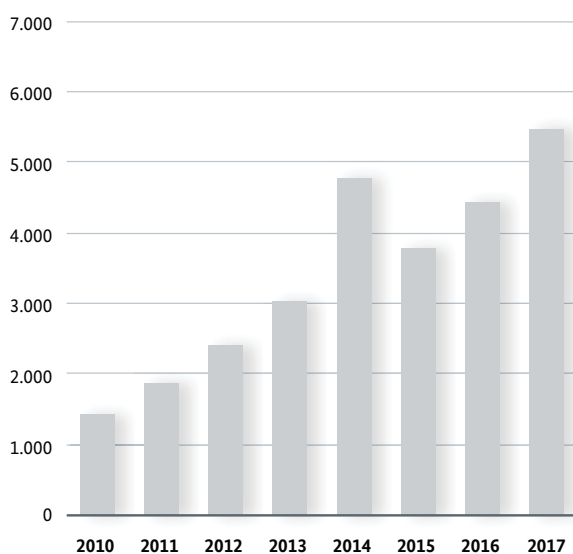
Abbildung 2: Jährlicher Leistungszubau in MW, Windenergie an Land seit 2010
