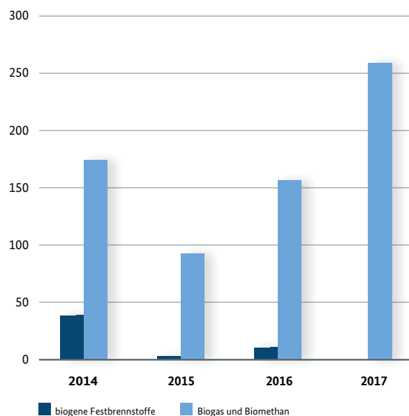
Abbildung 4: Jährlicher Leistungszubau in MW, für biogene Festbrennstoffe sowie Biogas/Biomethan
