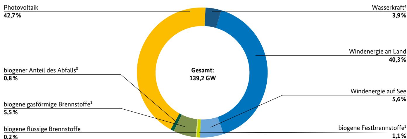
Abbildung 2: Aufteilung der installierten Leistung zur Stromerzeugung aus erneuerbaren Energien im Jahr 2021 nach Energieträgern
