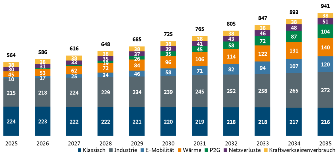
Interpolierter Stromverbrauch in Deutschland [TWh]
