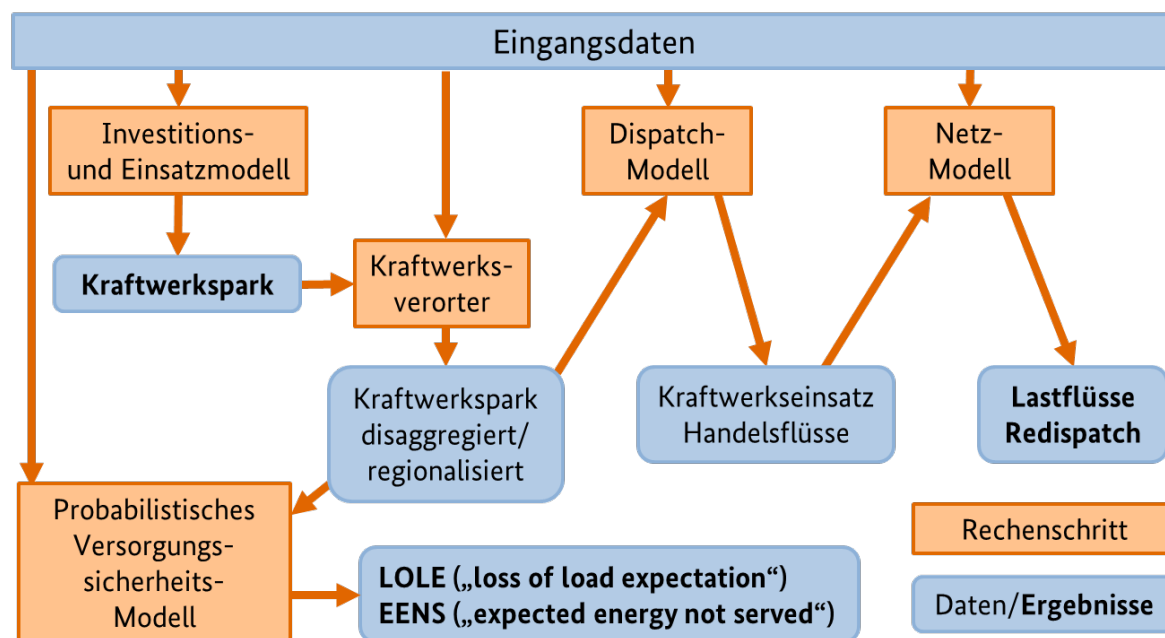
Abbildung 7: Übersicht Modellkette
