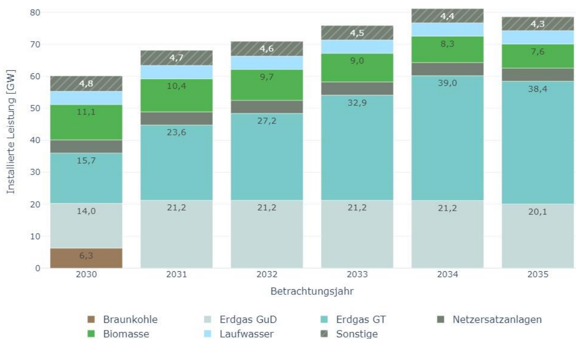
Abbildung 26: Installierte Leistung der Kraftwerke in Deutschland im VE-Szenario ohne Kraftwerksstrategie
