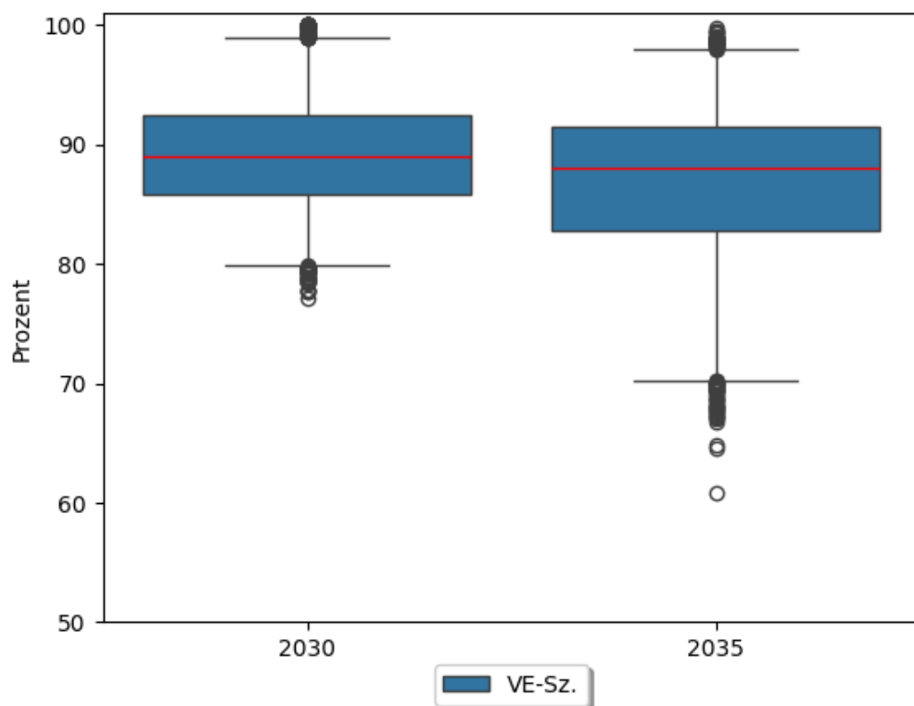
Abbildung 33: Relative Auslastung der Importkapazitäten im VE-Szenario 66
