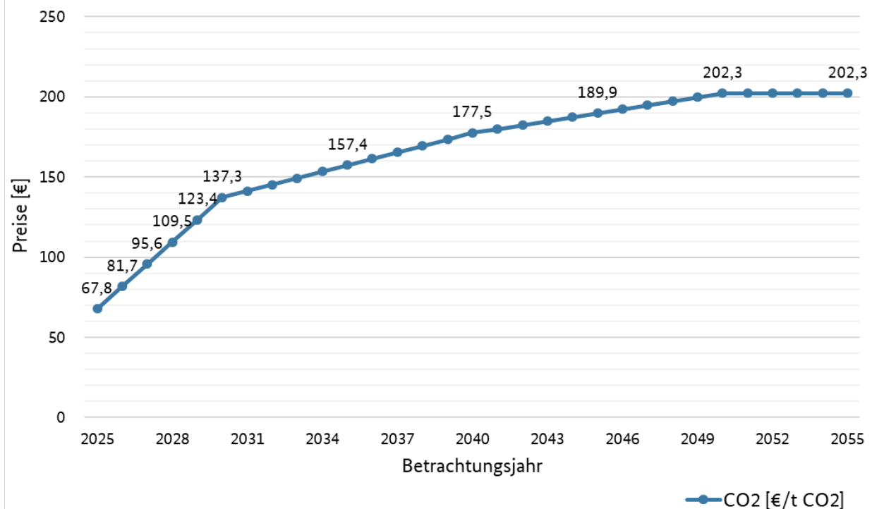
Abbildung 1: CO 2 -Zertifikate Preise; (Quelle: IEA)
