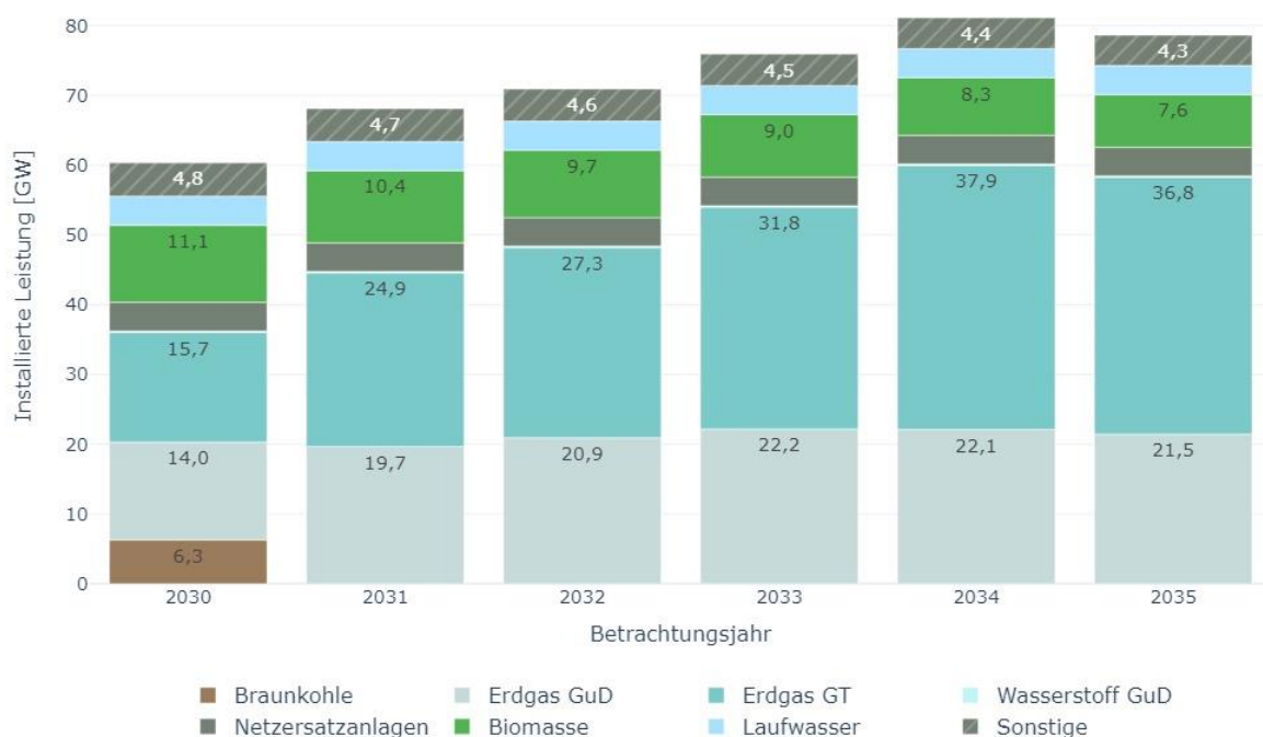
Abbildung 25: Installierte Leistung der Kraftwerke in Deutschland im VE-Szenario
