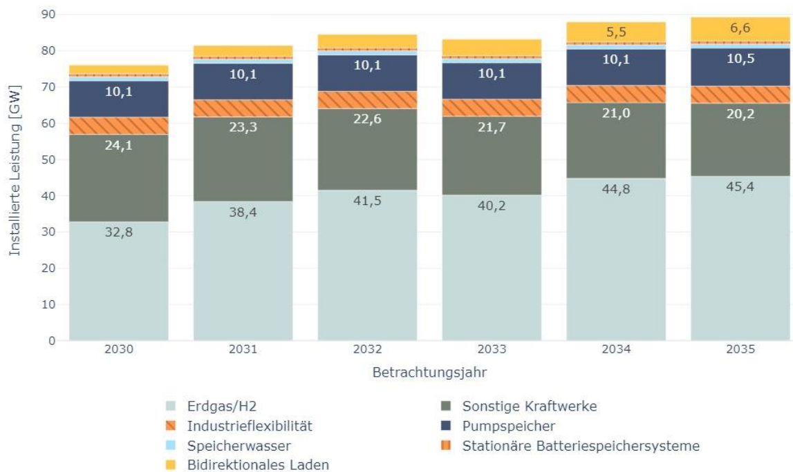
Abbildung 9: Entwicklung der steuerbaren Kapazitäten in Deutschland im Zielszenario
