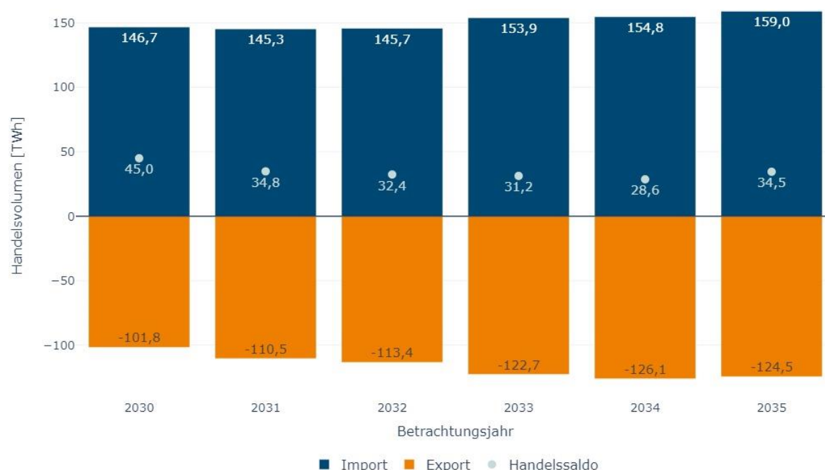
Abbildung 18: Stromhandelssaldo für die Gebotszone Deutschland-Luxemburg im Zielszenario
