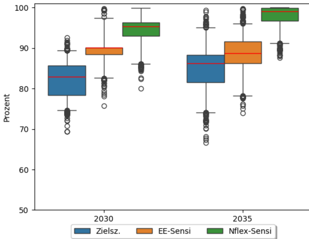
Abbildung 20: Relative Auslastung der Importkapazitäten im Zielszenario 55
