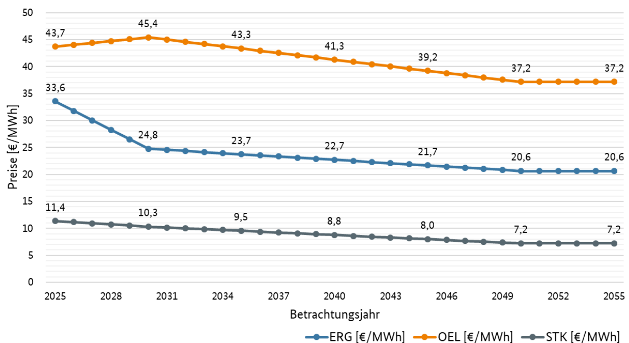
Abbildung 2: Brennstoffpreise; (Quelle: IEA)
