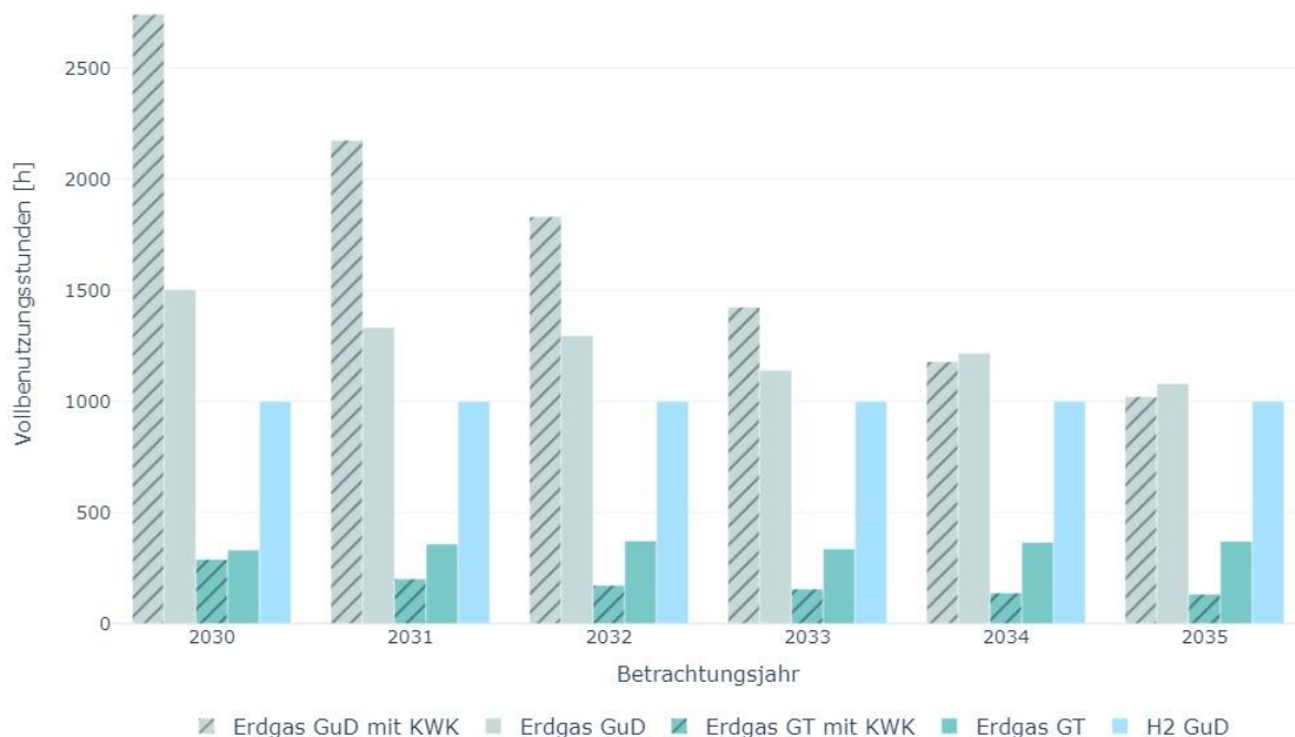
Abbildung 13: Vollbenutzungsstunden für Gaskraftwerke in Deutschland im Zielszenario
